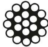
1x19 Monotron Teleferik Halatı
