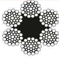
6x36 WS Kendir Öz (TS 1918/14)
