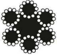
6x12 + 7 L.Öz Gergi Halatı
