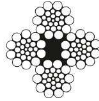
4x26 WS Trifor Halatı
