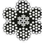
6x19 + (7x7) Ç.Öz Standart
