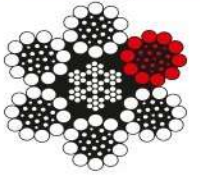
6x25 Ç.Öz WS FİLLER (TS 1918/11)
