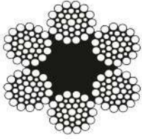
6x36 WS L.Öz (TS 1918/14)
