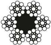
6x19 Seale Ağır Galvaniz (Balıkçılık Halatı)
