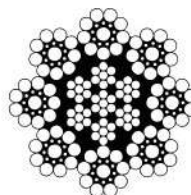
8x19 Seale Ç. Öz (Asansör Halatı)
