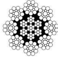
8x19 + (7x7) Seale Ç. Öz (TS 1918/18) Asansör Halatı
