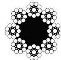
8x19 Seale L. Öz (Asansör Halatı)
