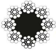
8x19 Seale L. Öz (TS 1918/18) Asansör Halatı
