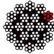
19x7 Ç. Öz (TS 1918/24) Nuflex Dönmeyen Halat
