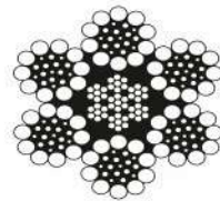
6x26 Ç. Öz WS FİLLER (TS 1918/11)
