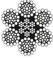
6x36 WS Çelik Öz (TS 1918/14)
